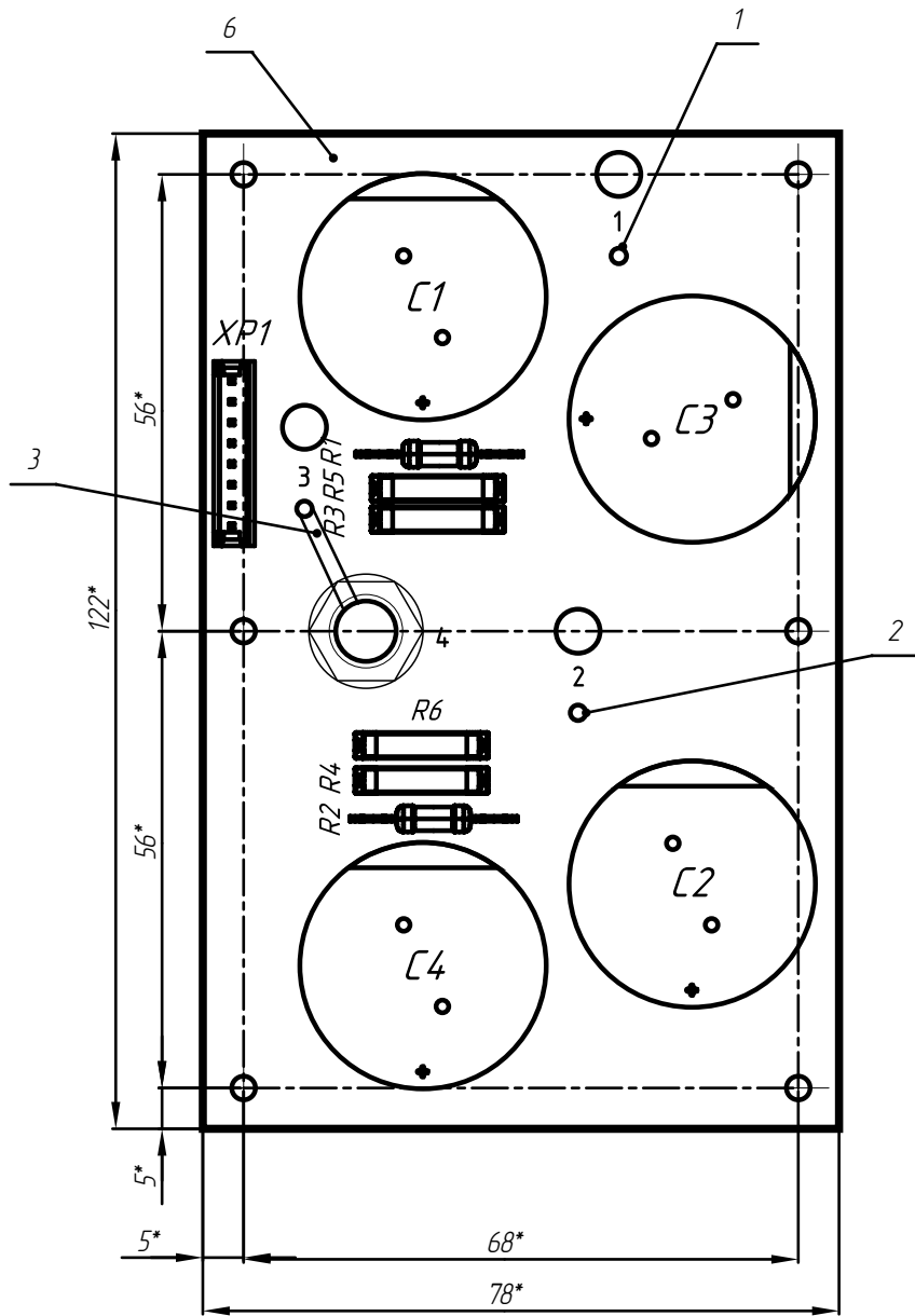
Установка проводов в т.1, 2.
